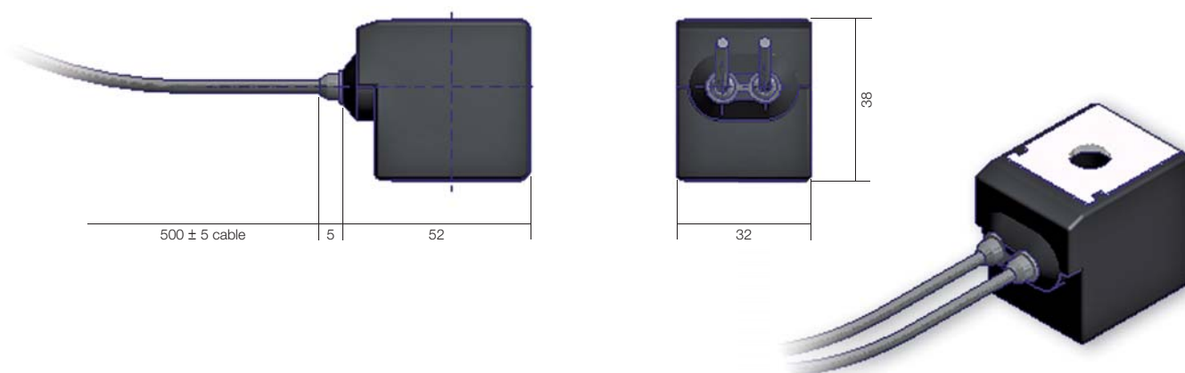
Plano de dimensiones Núm. 11
